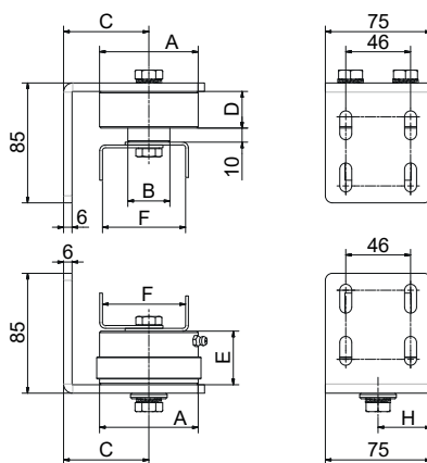
Modello depositato Materiale: Acciaio Zincato
