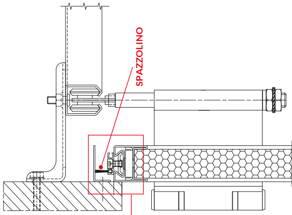
SOLUZIONE STANDARD parte superiore CON SPAZZOLINO
