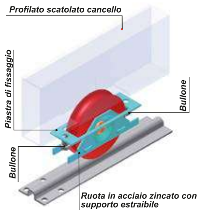
Ruote con piastra estraibile
